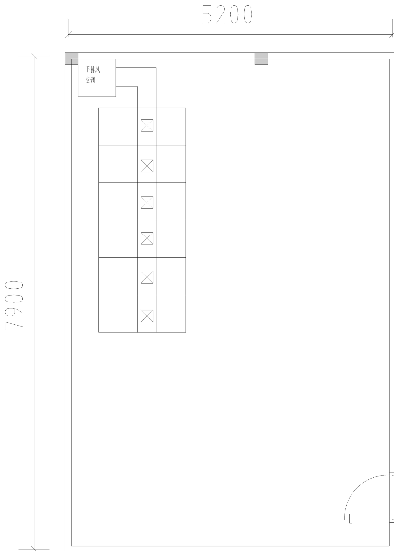
排风走向图
