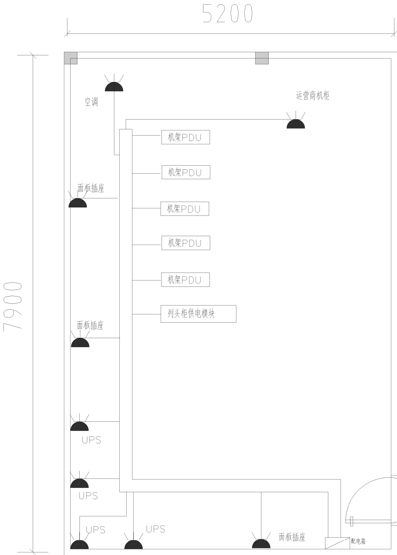
插座走向图
